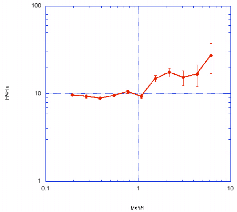
PHA_FLX_EVENT_4_R_4HE
