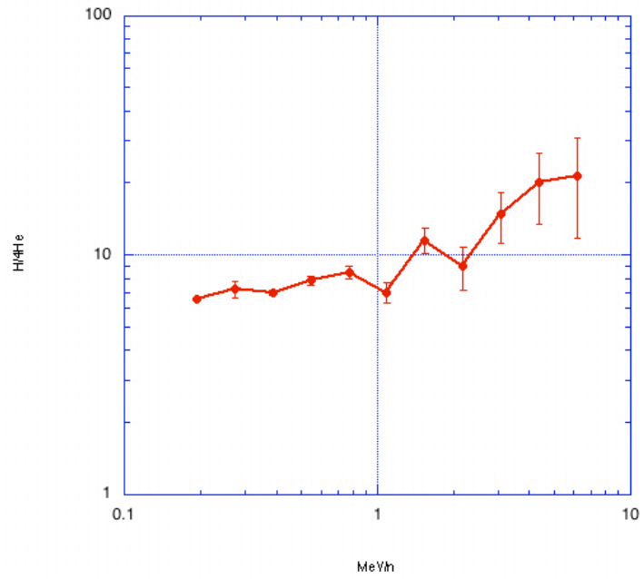
PHA_FLX_EVENT_3_R_4HE
