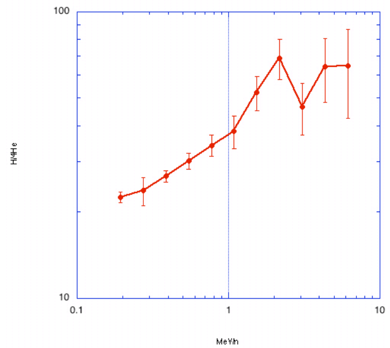
PHA_FLX_EVENT_2_R_4HE
