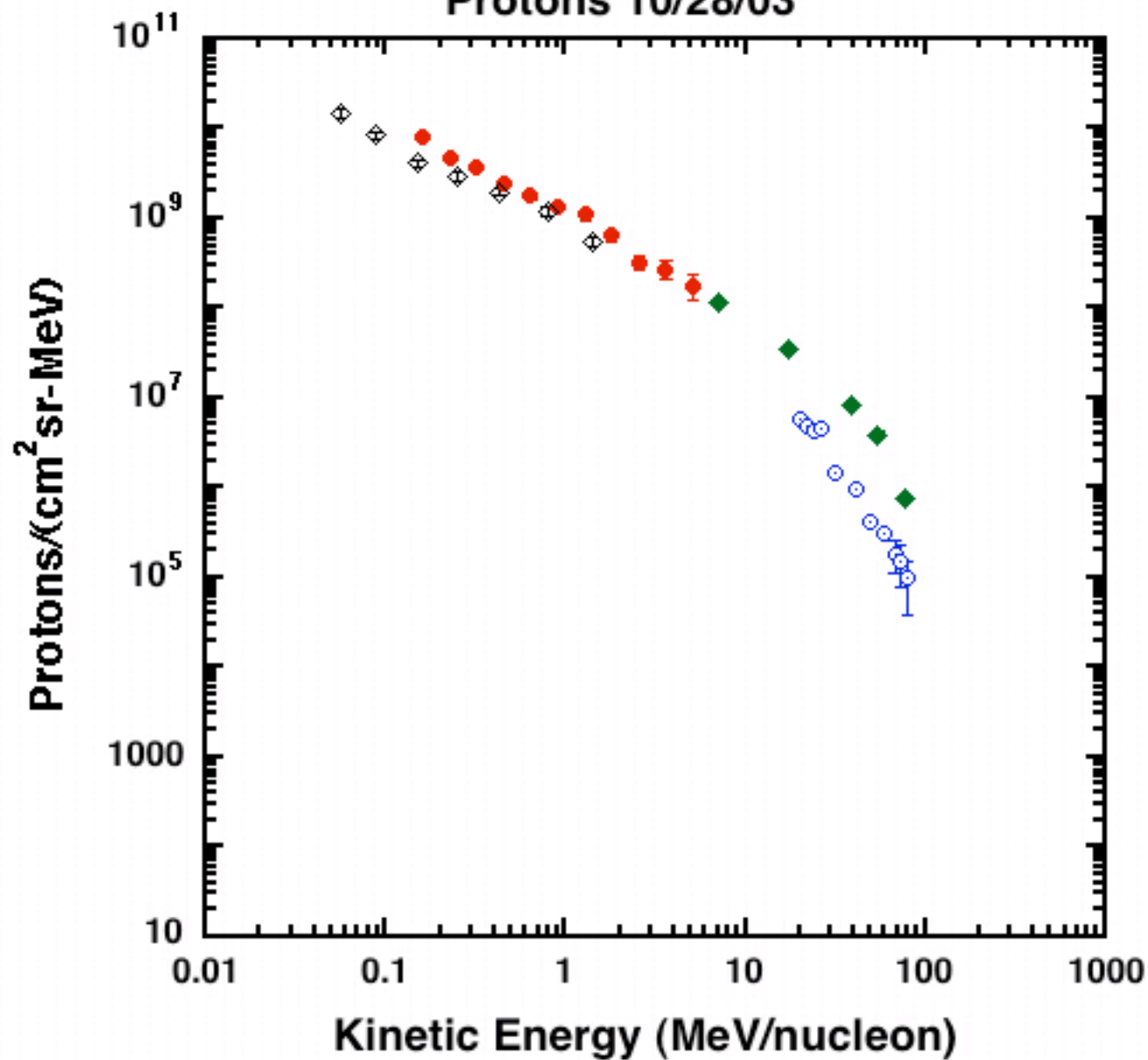
Protons 10/28/03
