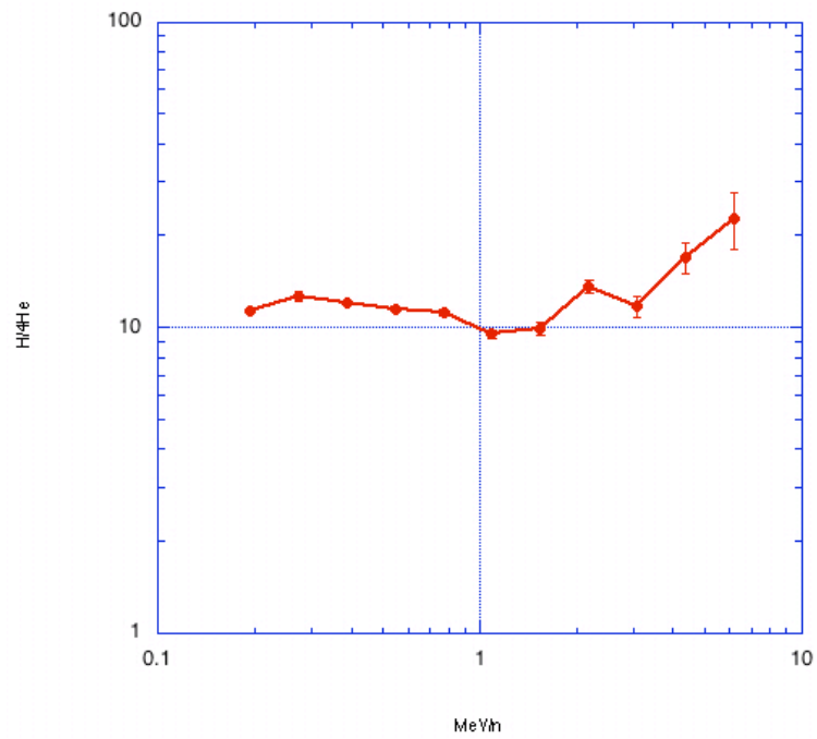
PHA_FLX_EVENT_1_R_4HE
