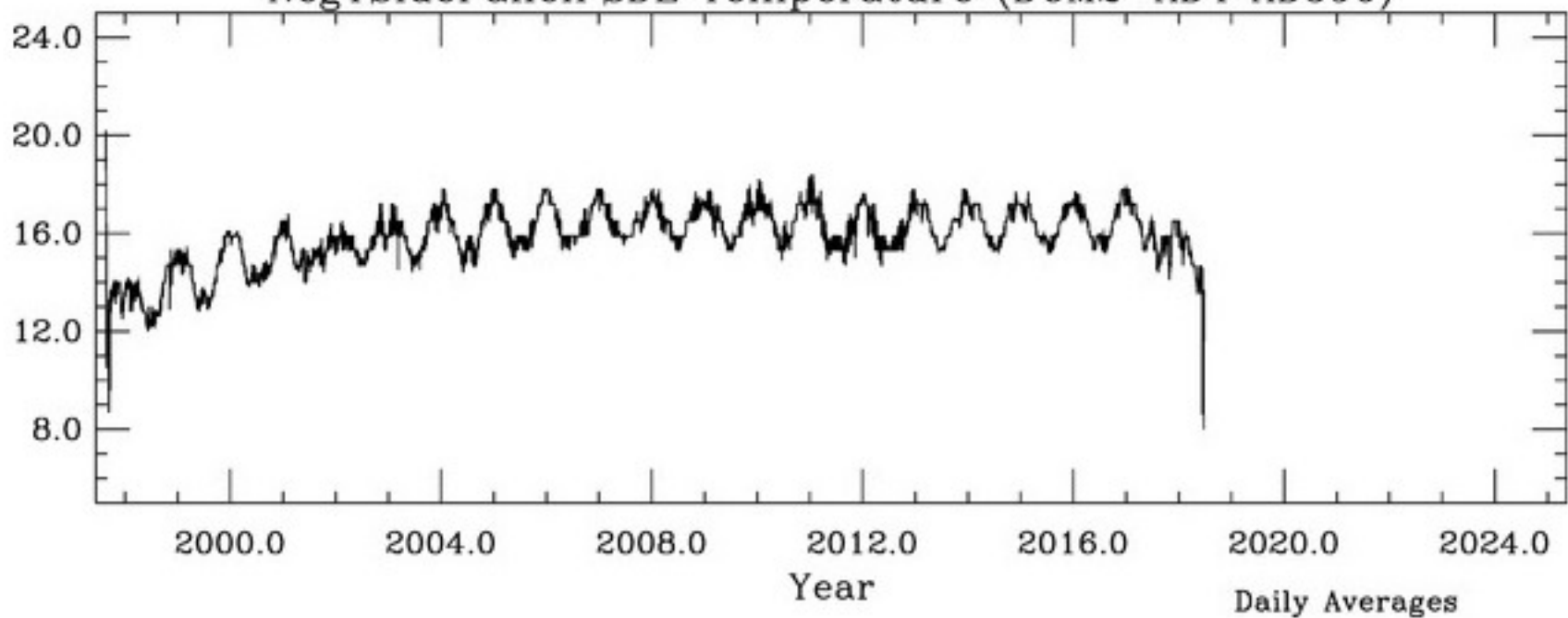
NegYSidePanelPSDE Temperature (DCM2-AD4 AD590)
