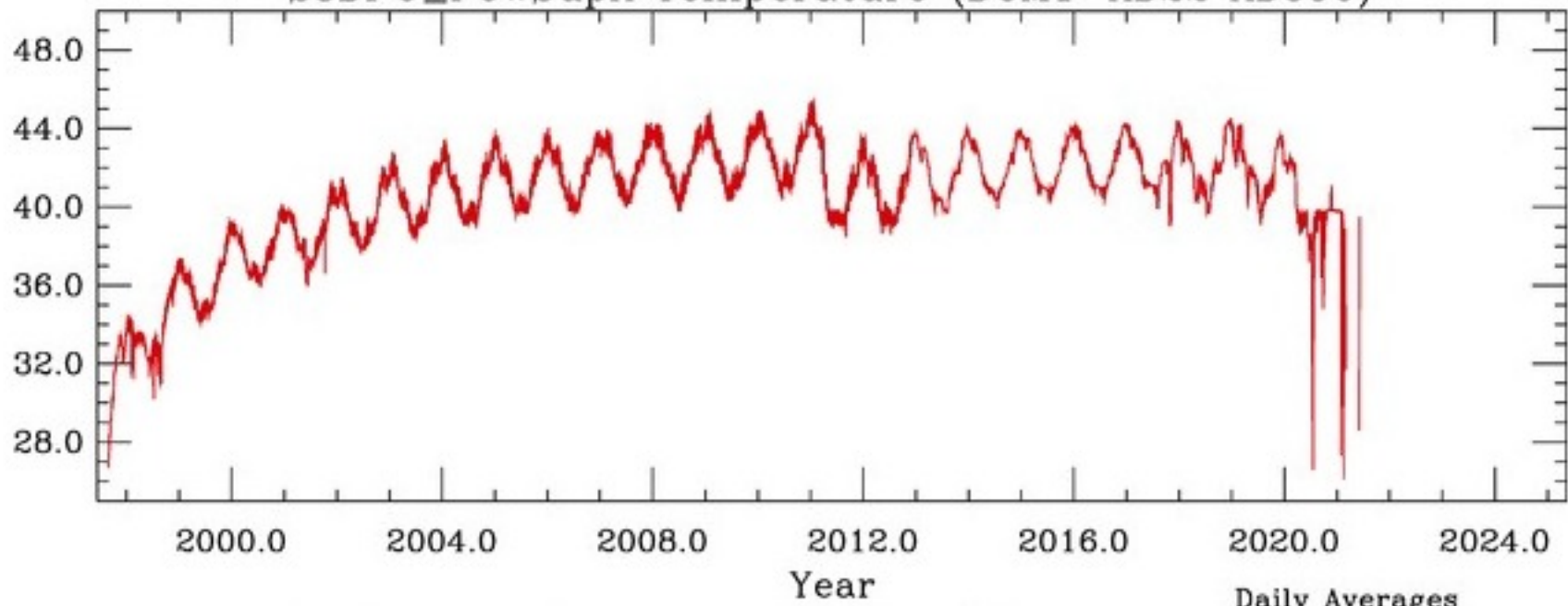
S3DPU_PowSupB Temperature (DCM1-AD30 AD590)
