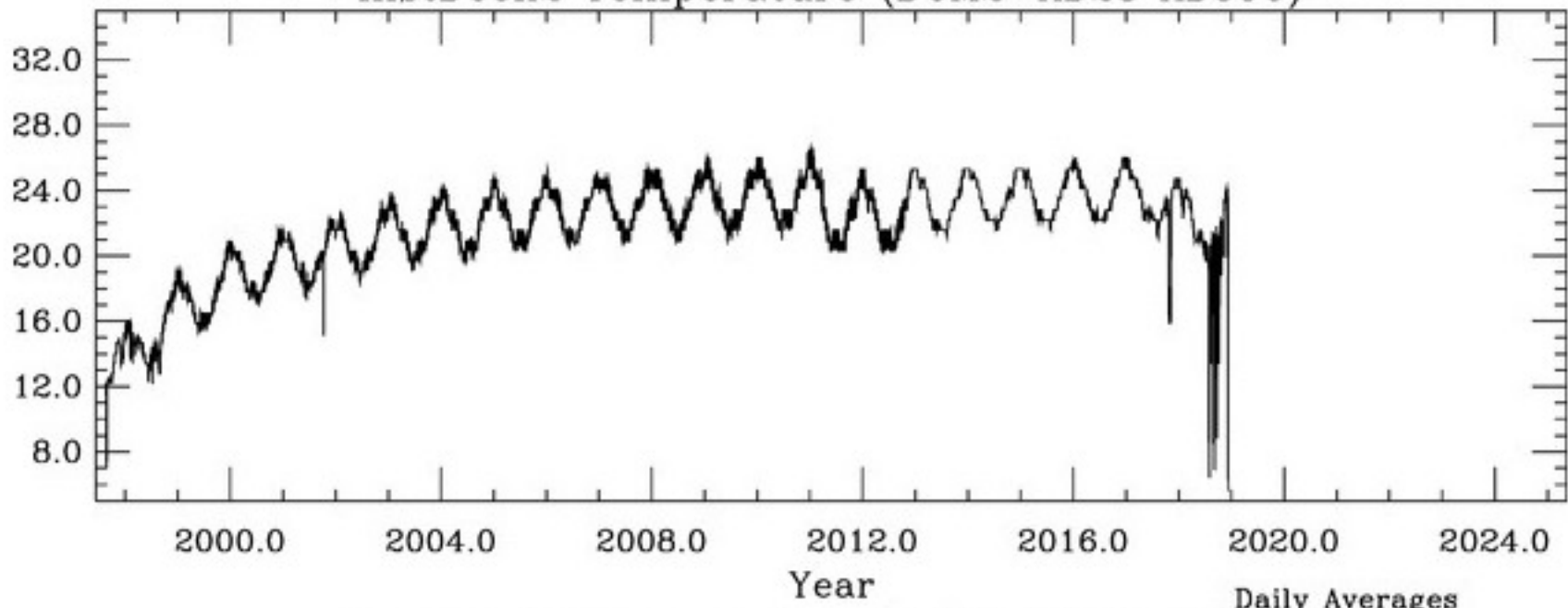
InstDeck3 Temperature (DCM2-AD24 AD590)
