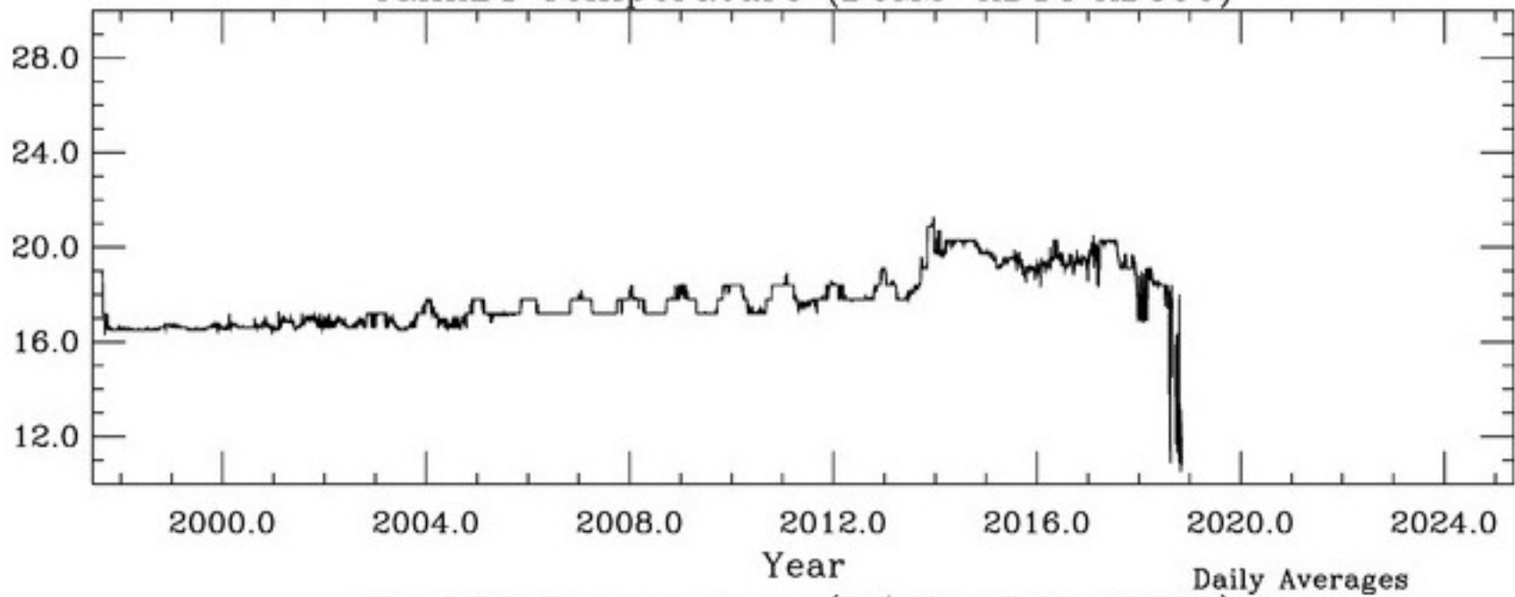
TankB2 Temperature (DCM2-AD15 AD590)
