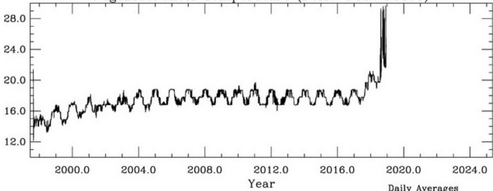
NegYSidePanelPSDE Temperature (DCM2-AD4 AD590)
