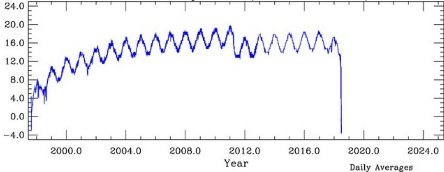
InstDeck4 Temperature (DCM2-AD25 AD590)
